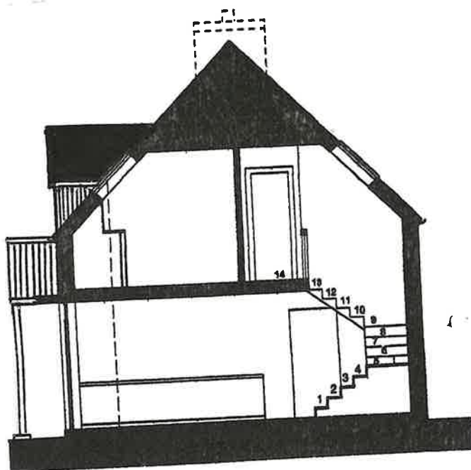
SECTION DD
