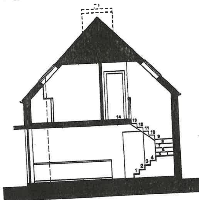
SECTION DD
